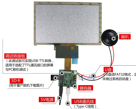
图 1-4 调试工具图
