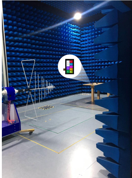
图 6-4 RE 测试图
