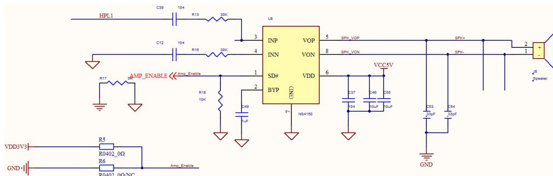
图 3-3 音频参考电路
