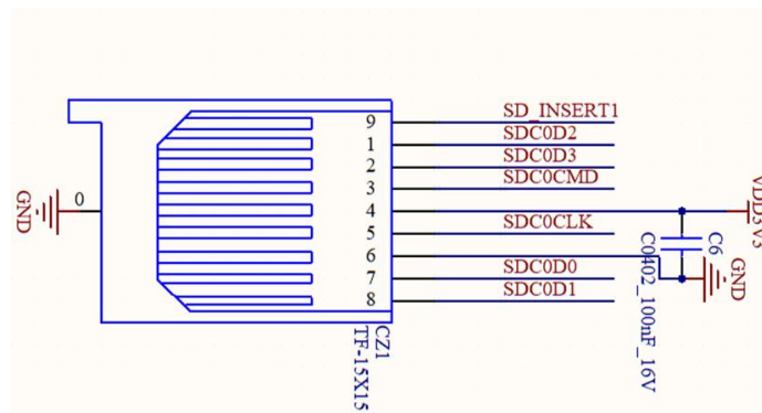
图 3-2 SD 卡参考电路
