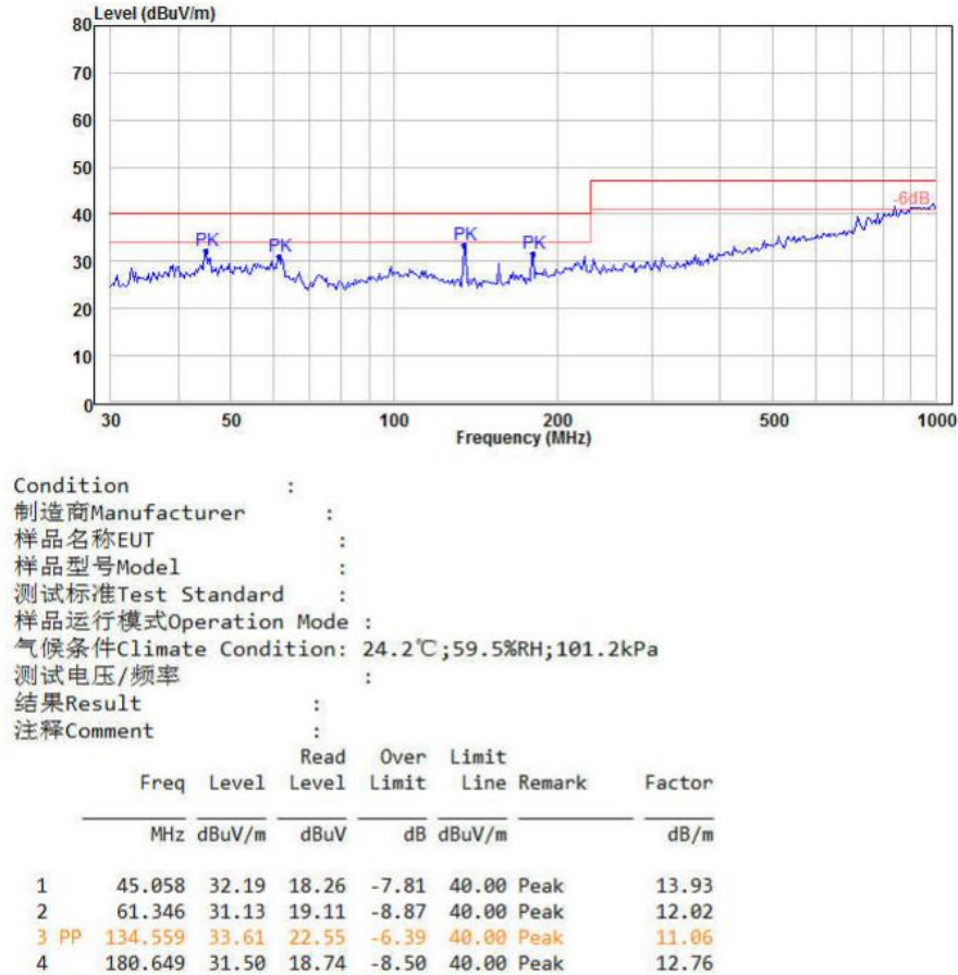
图 6-6 RE 测试垂直方向
