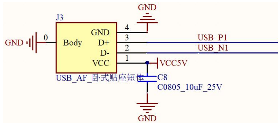
图 3-5 U 盘参考电路
