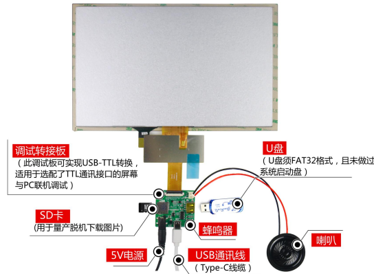
图 1-3 硬件配置图
